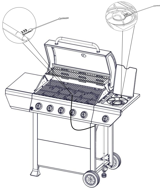
Quemador principal
