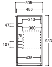
【共通側面図】
