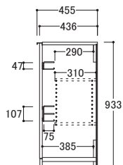
【共通側面図】
