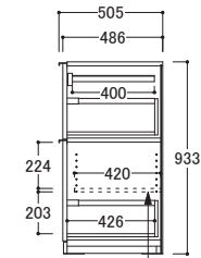
【側面図】
