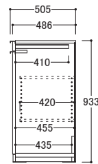
【共通側面図】
