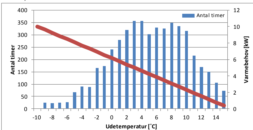
Figur 1: Eksempel på temperaturfordeling og varmebehov for en varmesæson
