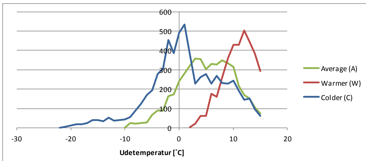
Figur 2: Fordeling af temperaturer for de tre klimazoner Average, Warmer og Colder
