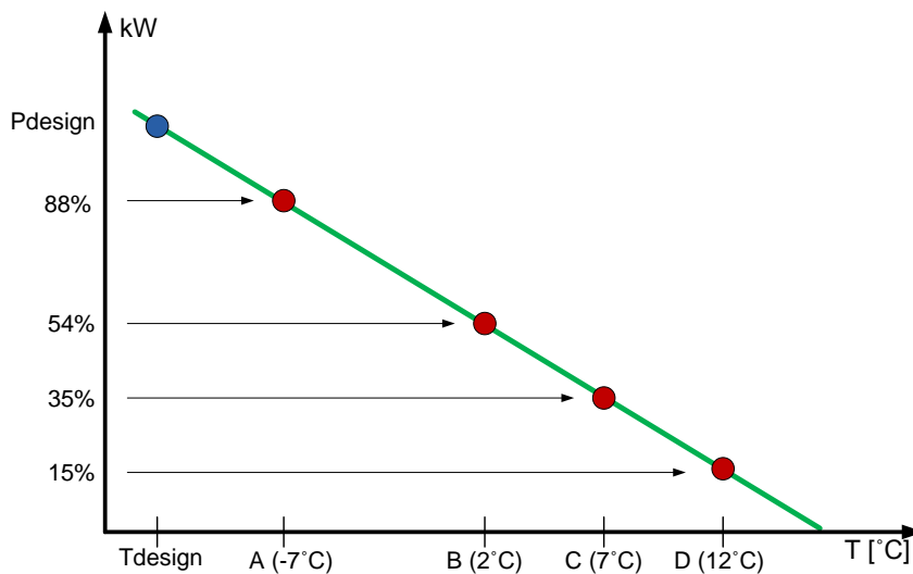
Figur 4: Definition af varmebehovskurven ud fra P_{design,h}
