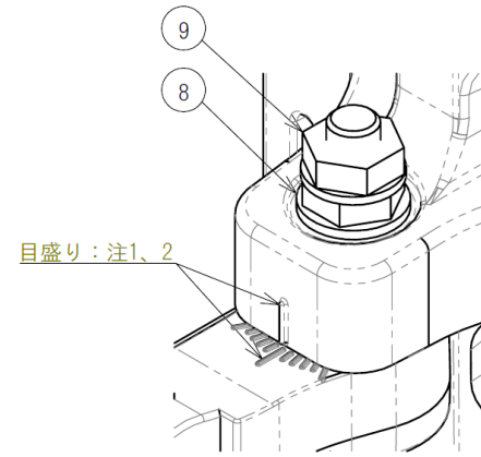
詳細図 FIG. A スケール 1 : 1
