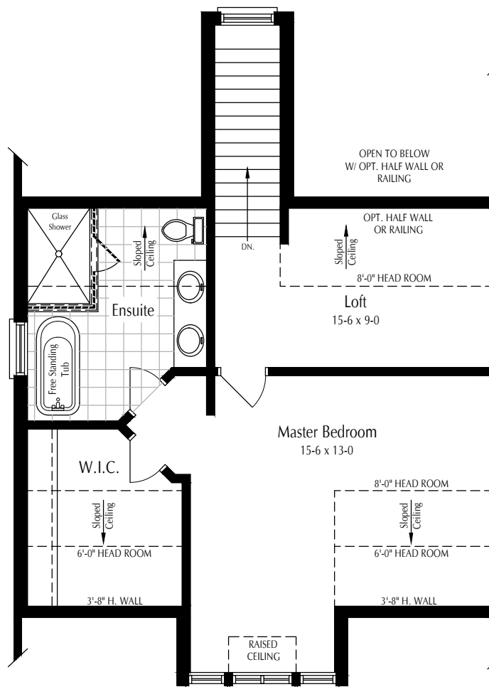
OPTIONAL LOFT PLAN 721 SQ.FT.
