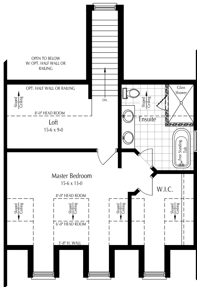
OPTIONAL LOFT PLAN 731 SQ.FT.
