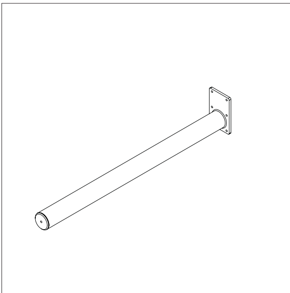
BOOM - D2-ix L x Ø: 800 x Ø60
