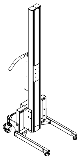
200 L/M/H FC - Flexleg type 1
