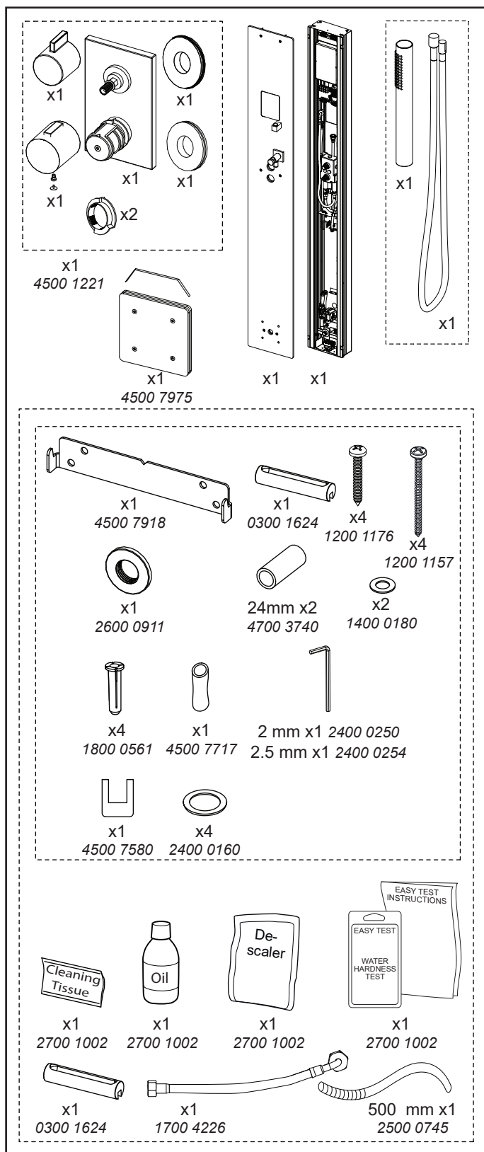
Kuva 1 Höyrypylvään osat
