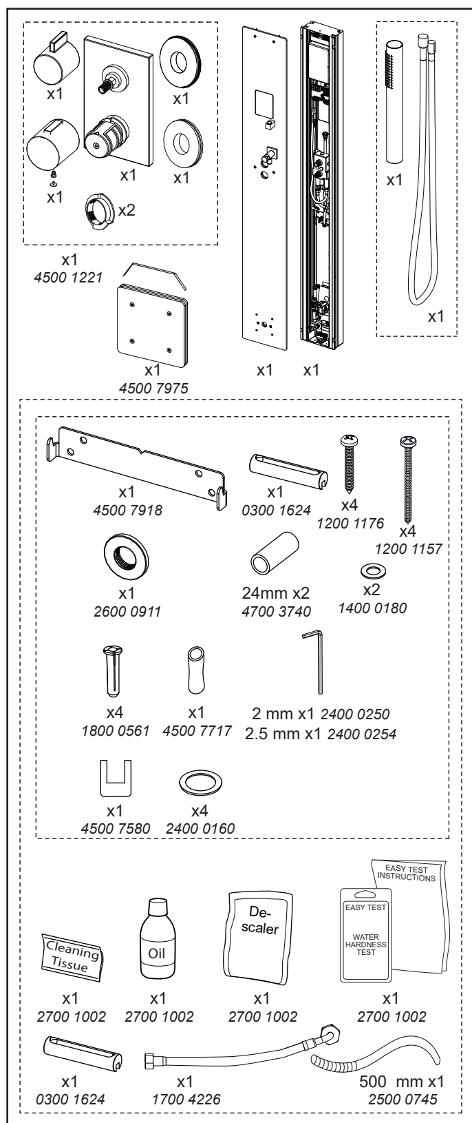
Afb. 1 Stoomkolom onderdelen
